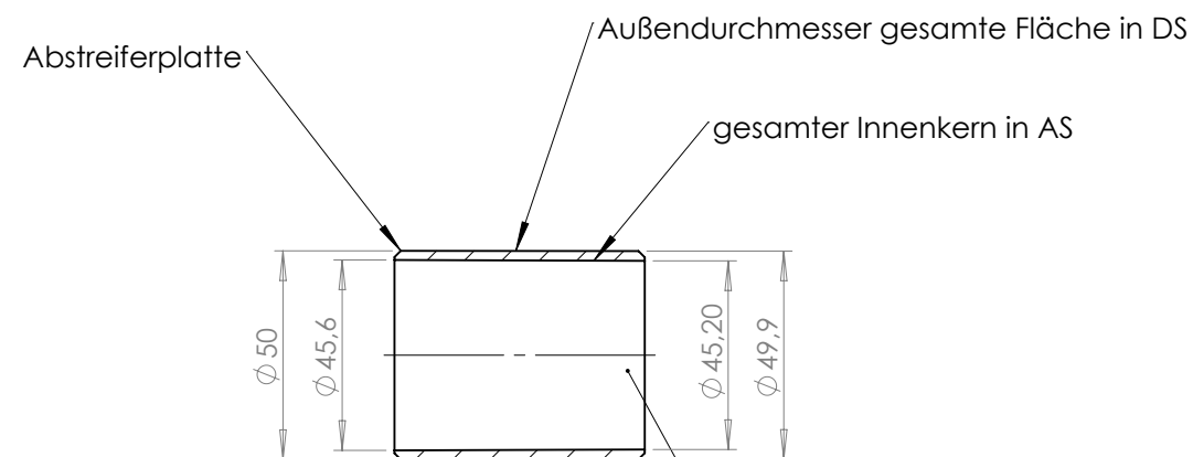
SCHNITT A-A Tunnelanguss 3 x \varnothing 2,5
