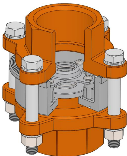
Mit montierten Stutzen für Gewindeanschlüsse (Typ 933)
