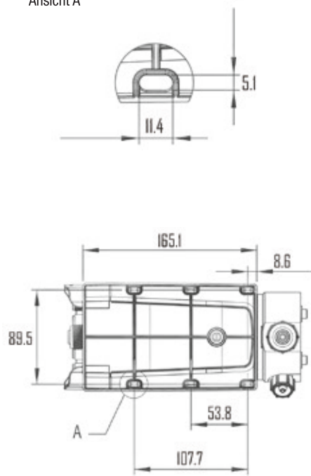
Ansicht A
